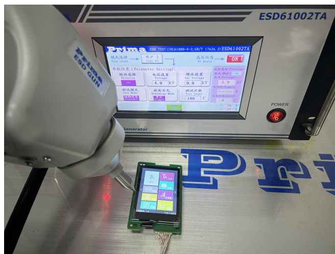
图 5-2 ESD 测试图
