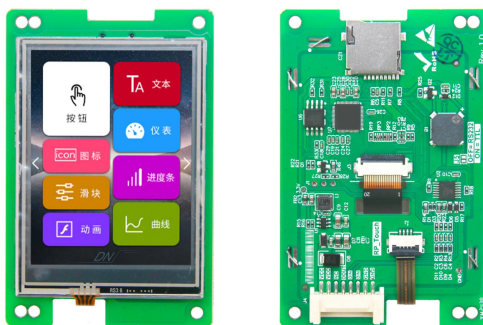
图 1-1 2.8 寸电阻触摸参考图
