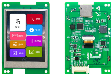
图 1-3 2.8 寸无触摸参考图
