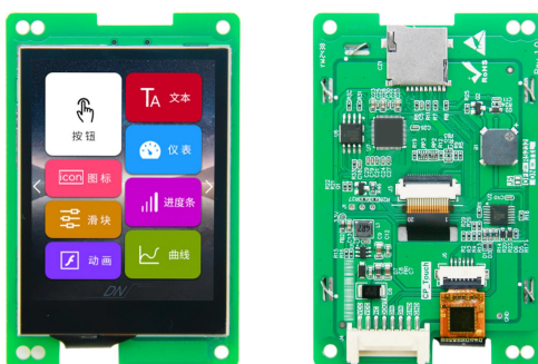
图 1-2 2.8 寸电容触摸参考图
